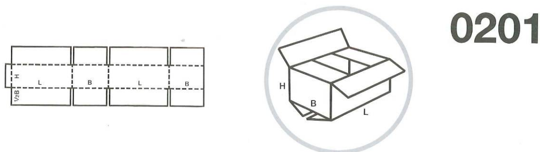
Abb. 1: Faltschachtel gemäß FEFCO 0201
