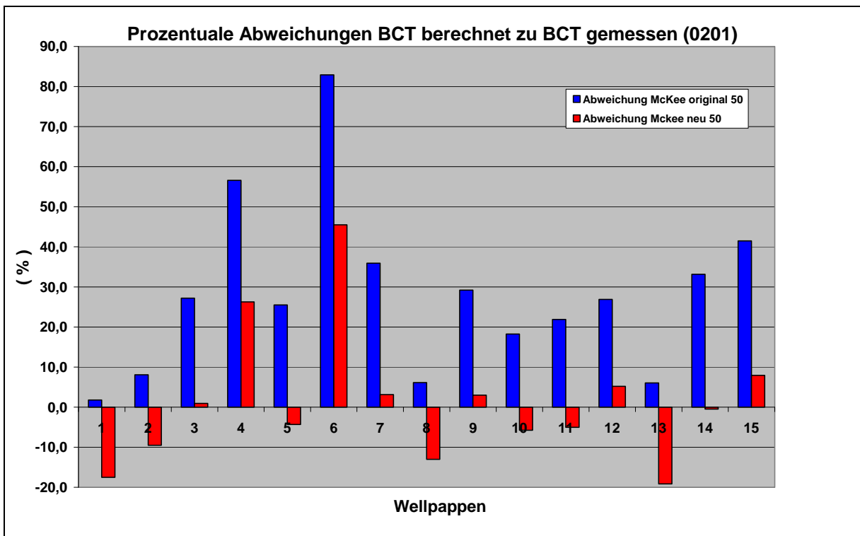
Abb. 13: Prozentuale Abweichungen zwischen BCT berechnet und BCT gemessen (alt/neu), Packmittel FEFCO 0201 bei 50 % rel. LF.
